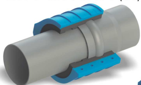
Cabezal Cubre Cabeza (CC)
